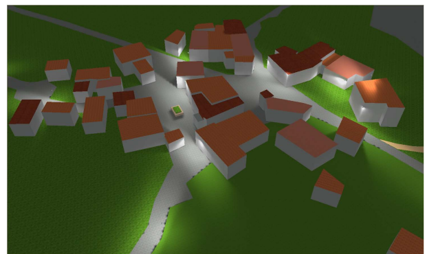
Simulación de la iluminación con LED en Momediano
